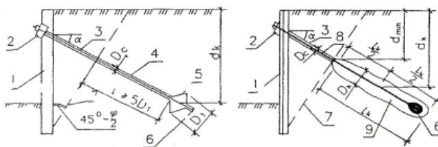
Рисунок M.1 - Схемы анкеров
