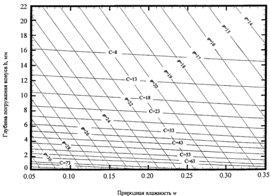
Рисунок Е.7 - Номограмма для определения удельного сцепления c_n , кПа, и угла внутреннего трения \rho , град., ледниковых (моренных) глинистых грунтов
