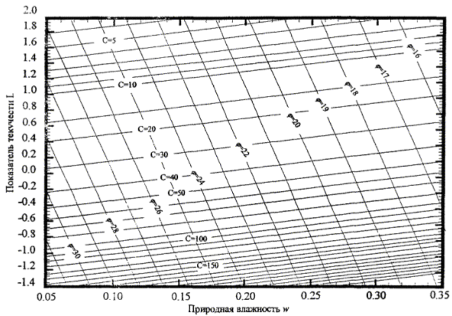
Рисунок Е.2 - Номограмма для определения сцепления c_n , кПа и угла внутреннего трения \varphi_n , град., ледниковых (моренных) глинистых грунтов
